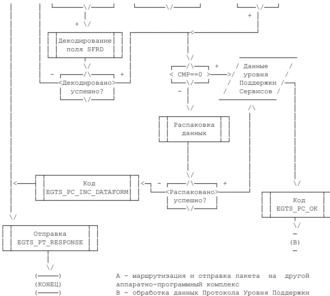
Рисунок 2. Блок-схема алгоритма обработки пакета данных протокола Транспортного уровня при приеме
