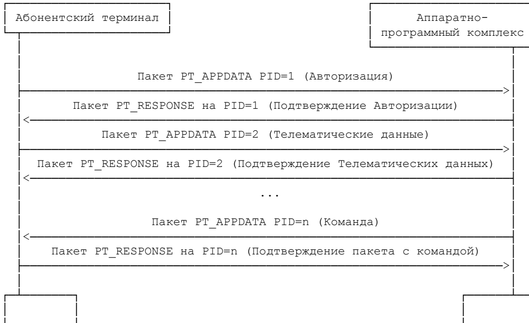
Рисунок N 3. Взаимодействие абонентского терминала и аппаратно-программного комплекса на уровне пакетов Транспортного уровня
